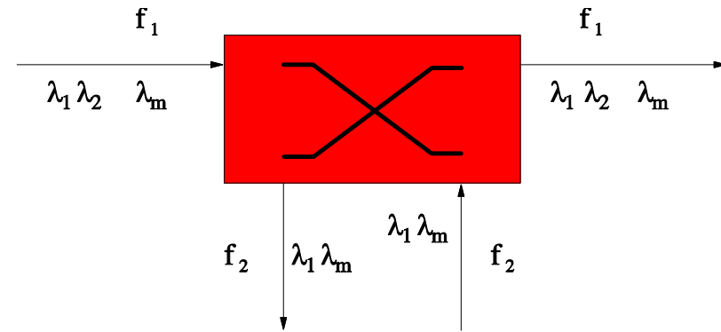
OADM
